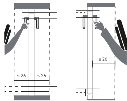
Laibungstiefe \leq 26
