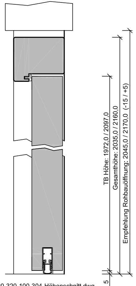
220-320-100-304-Höhenschnitt.dwg
