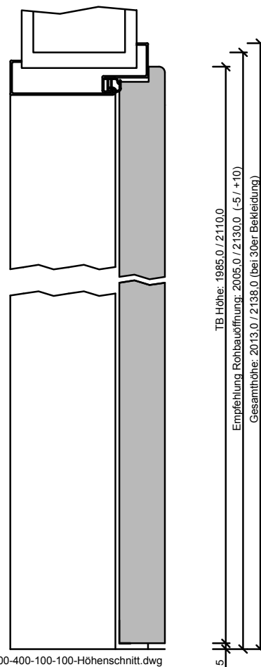
100-400-100-100-Höhenschnitt.dwg
