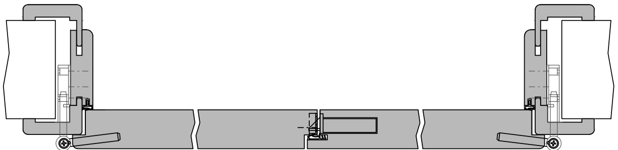
100-100-100-100-Höhenschnitt.dwg
