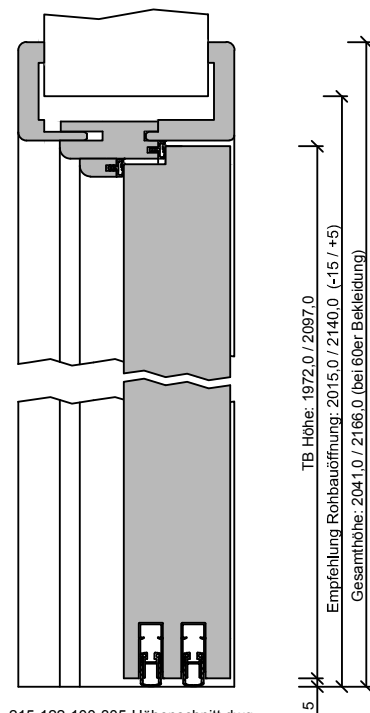
215-122-100-305-Höhenschnitt.dwg
