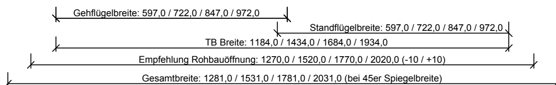
200-800-400-100-Querschnitt 2-flg.dwg
