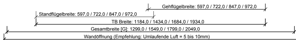
Q_RD_TB-BLO-2FLG_STU_RD-40-LA.dwg
