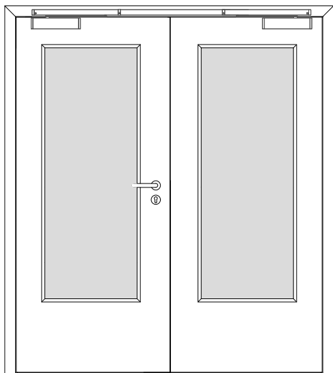
401-406-103-100_Ansicht.dwg
