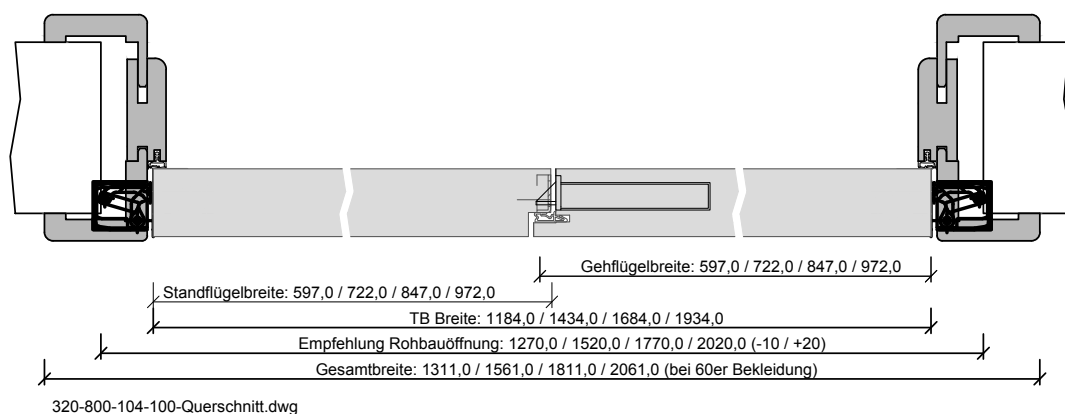
320-800-104-100-Querschnitt.dwg
