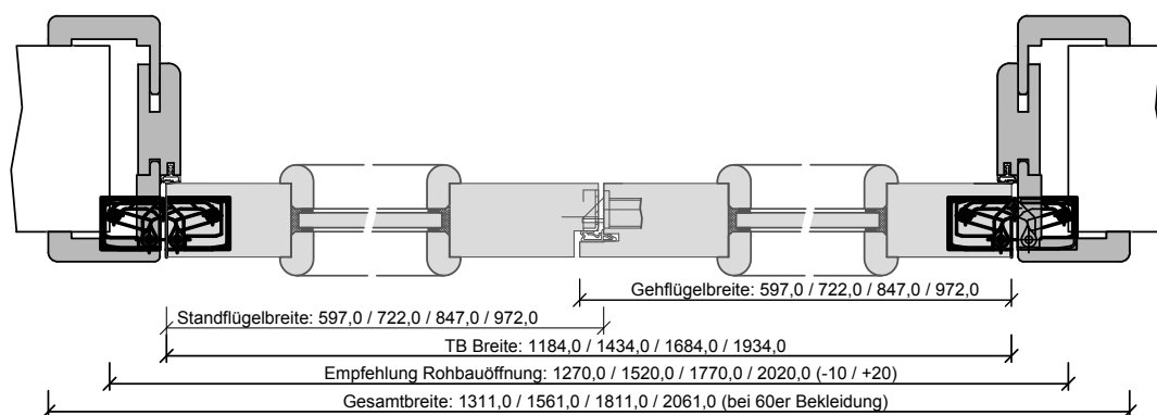
321-800-104-100-Querschnitt.dwg
