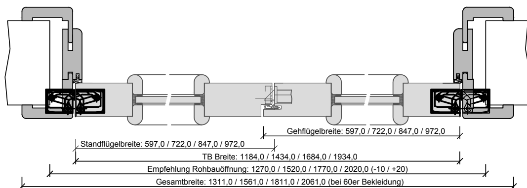
321-800-104-100-Querschnitt.dwg
