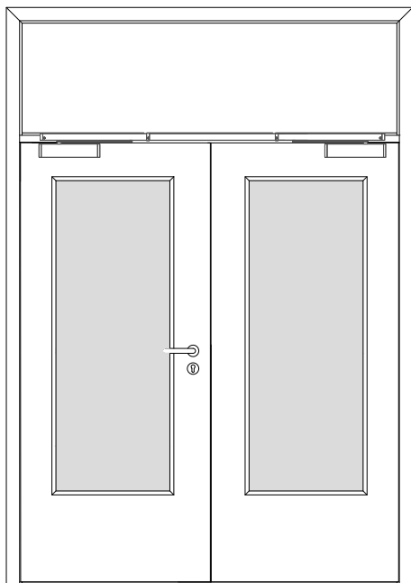
401-408-103-200_Ansicht.dwg
