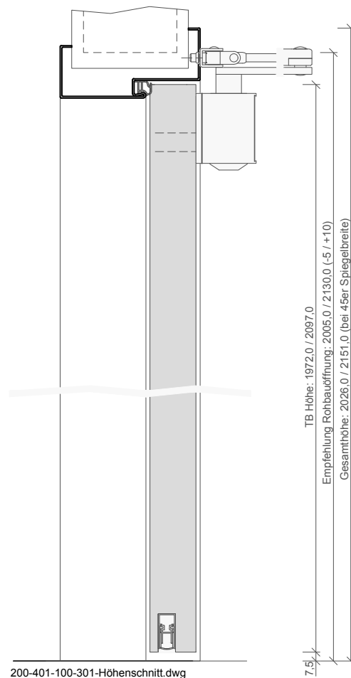
200-401-100-301-Höhenschnitt.dwg
