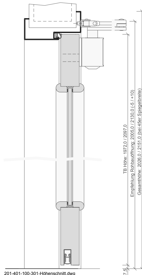
201-401-100-301-Höhenschnitt.dwg
