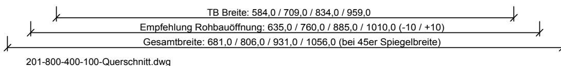
201-800-400-100-Querschnitt.dwg
