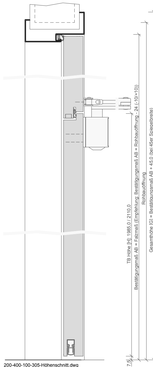
200-400-100-305-Höhenschnitt.dwg
