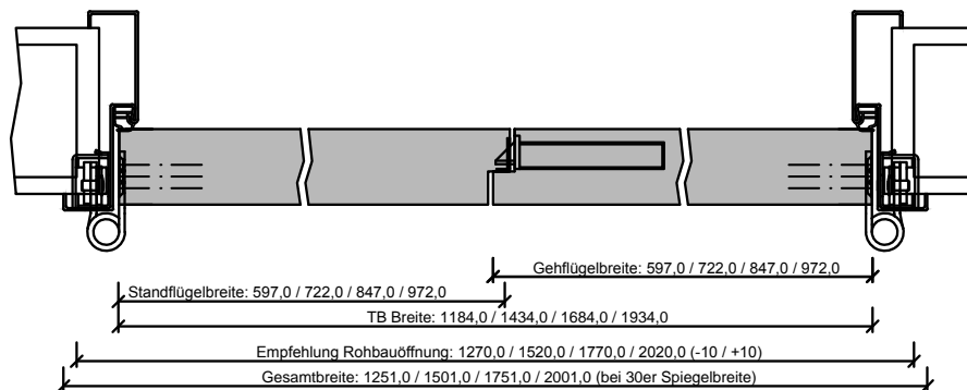
135-223-401-100-Querschnitt.dwg
