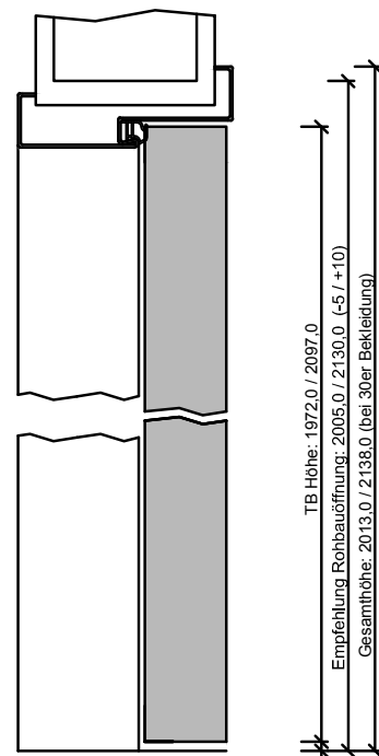
220-420-100-100-Höhenschnitt.dwg
