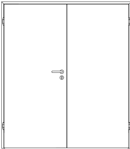
400-101-402-100_Ansicht.tcd
