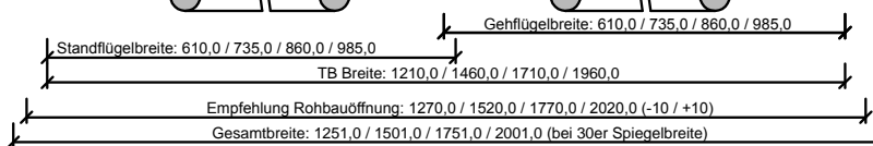
134-107-401-100-Querschnitt.dwg
