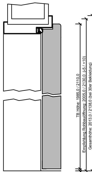
150-440-100-100-Höhenschnitt.dwg
