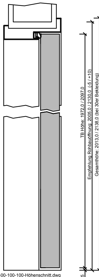
200-400-100-100-Höhenschnitt.dwg
