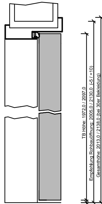
220-420-100-100-Höhschnitt.dwg
