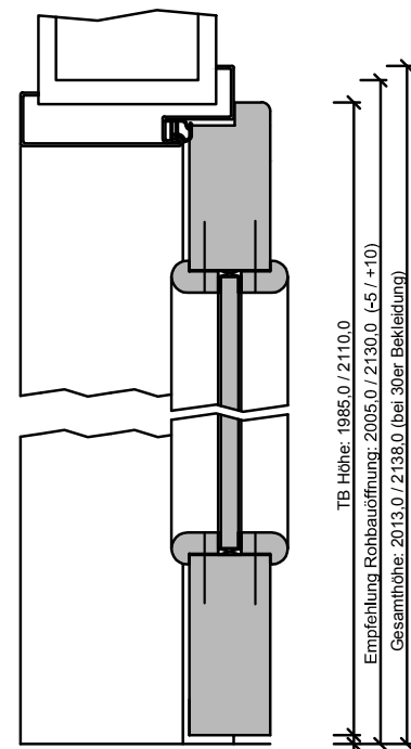
106-400-100-100-Höhenschnitt.dwg
