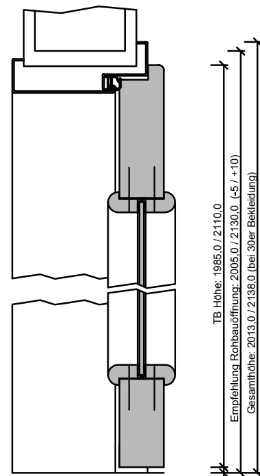
500-400-100-100-Höhenschnitt.dwg
