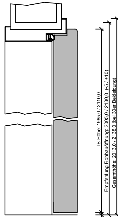
150-440-100-100-Höhenschnitt.dwg
