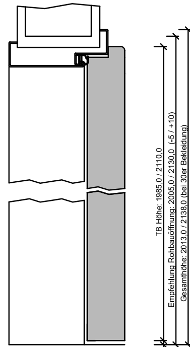
150-440-100-100-Höhenschnitt.dwg
