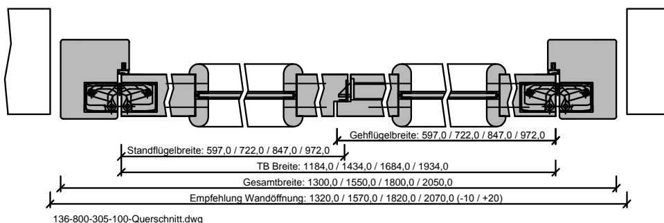
136-800-305-100-Querschnitt.dwg
