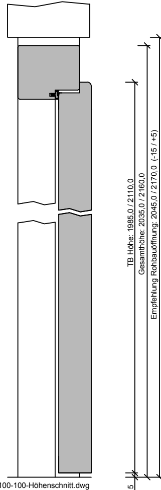
100-300-100-100-Höhenschnitt.dwg
