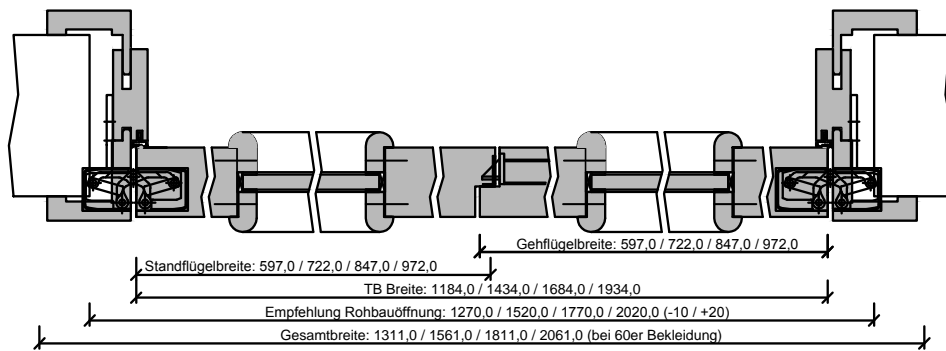
137-800-112-100-Querschnitt.dwg
