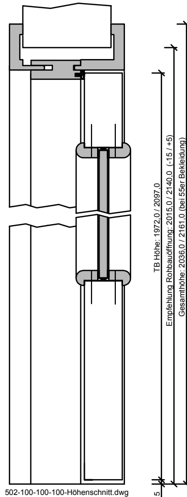
502-100-100-100-Höhenschnitt.dwg
