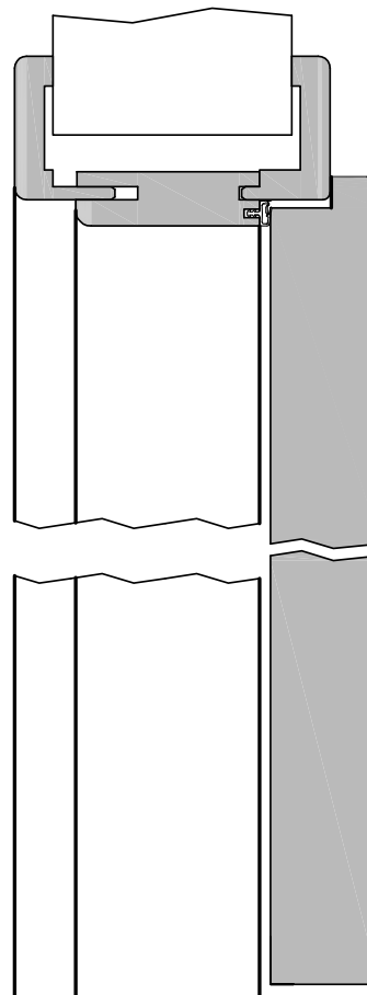
120-130-100-100-Höhenschnitt.dwg
