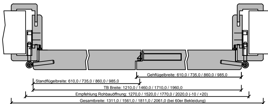
132-102-105-100-Querschnitt.dwg
