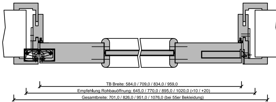
224-800-112-100-Querschnitt.dwg
