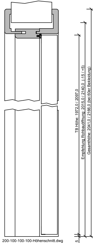
200-100-100-100-Höhenschnitt.dwg
