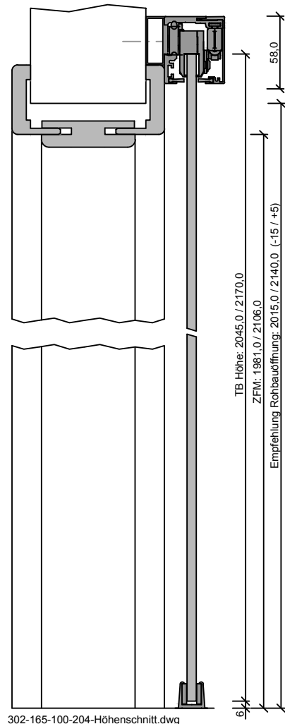
302-165-100-204-Höhenschnitt.dwg
