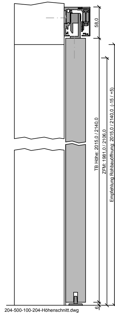
204-500-100-204-Höhenschnitt.dwg
