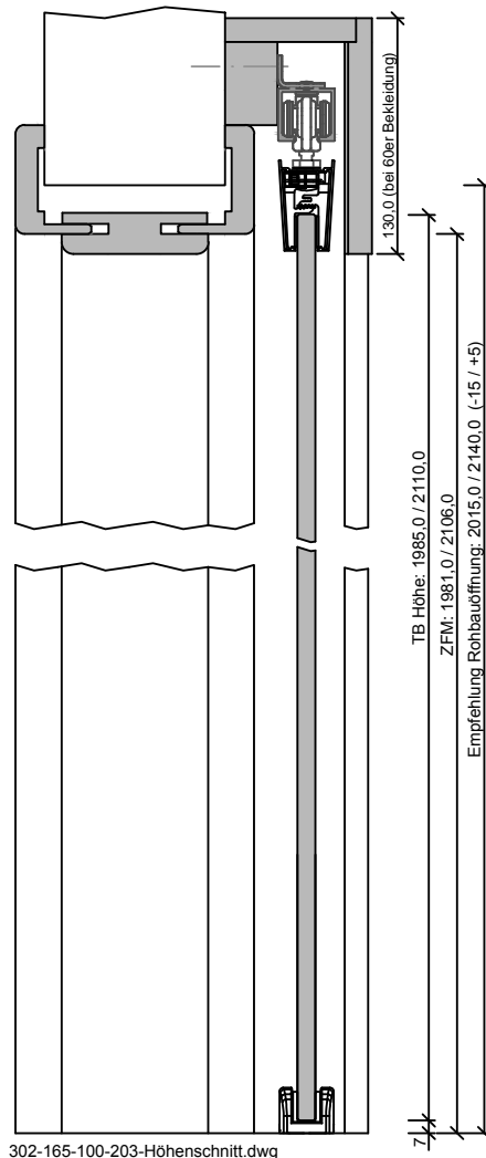
302-165-100-203-Höhenschnitt.dwg
