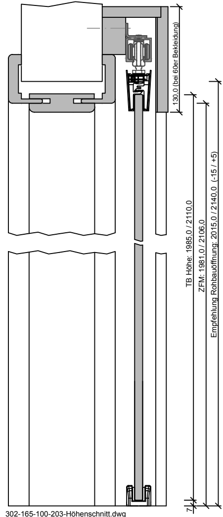
302-165-100-203-Höhenschnitt.dwg
