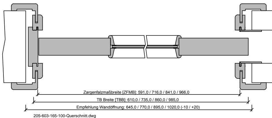
205-603-165-100-Querschnitt.dwg
