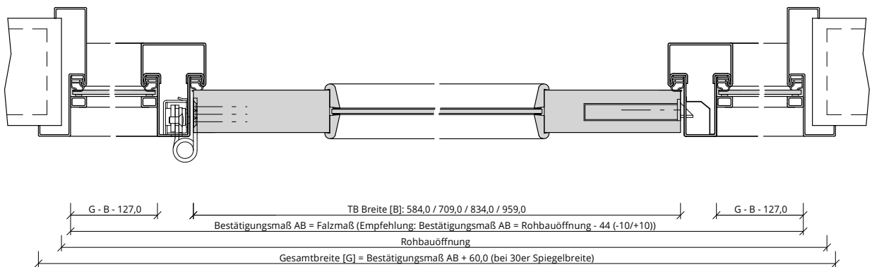
201-223-400-102-Querschnitt.tcd
