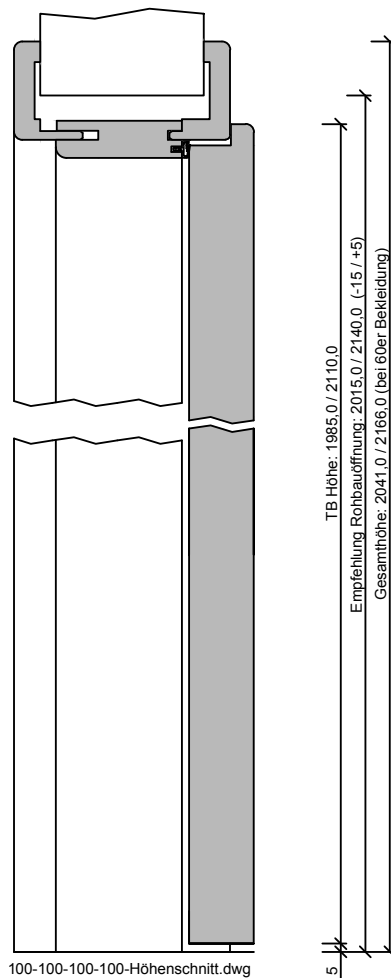
100-100-100-100-Höhenschnitt.dwg
