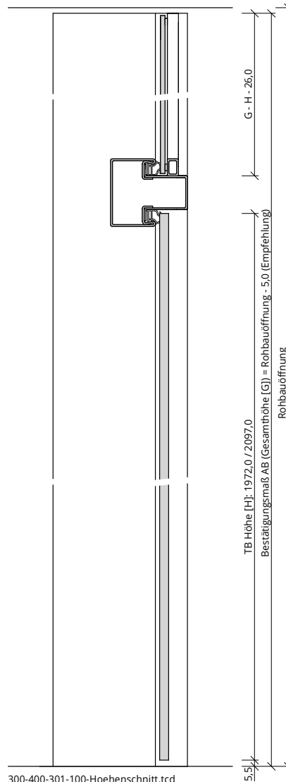
300-400-301-100-Hoehenschnitt.tcd
