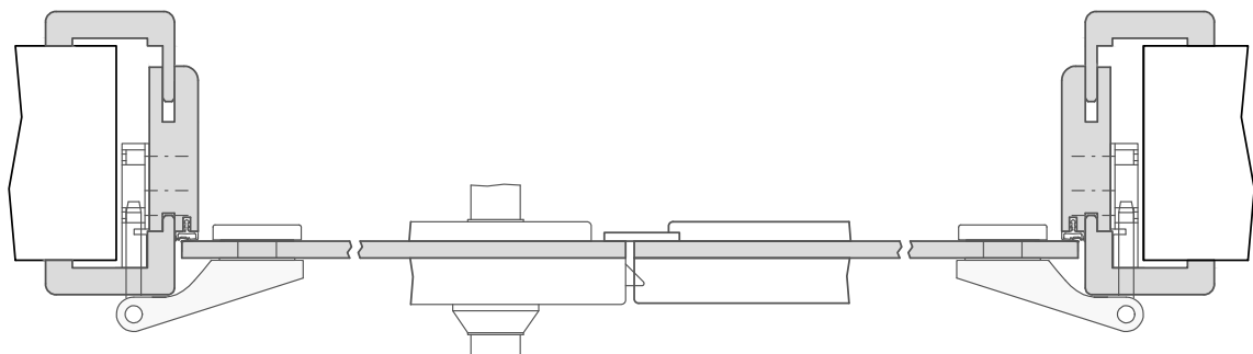
300-100-301-100-Höhenschnitt.dwg
