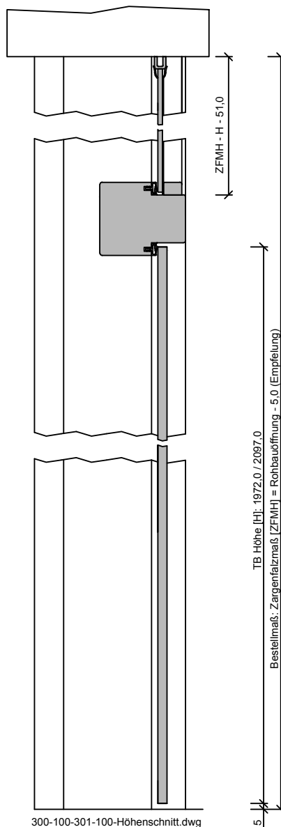
300-100-301-100-Höhenschnitt.dwg
