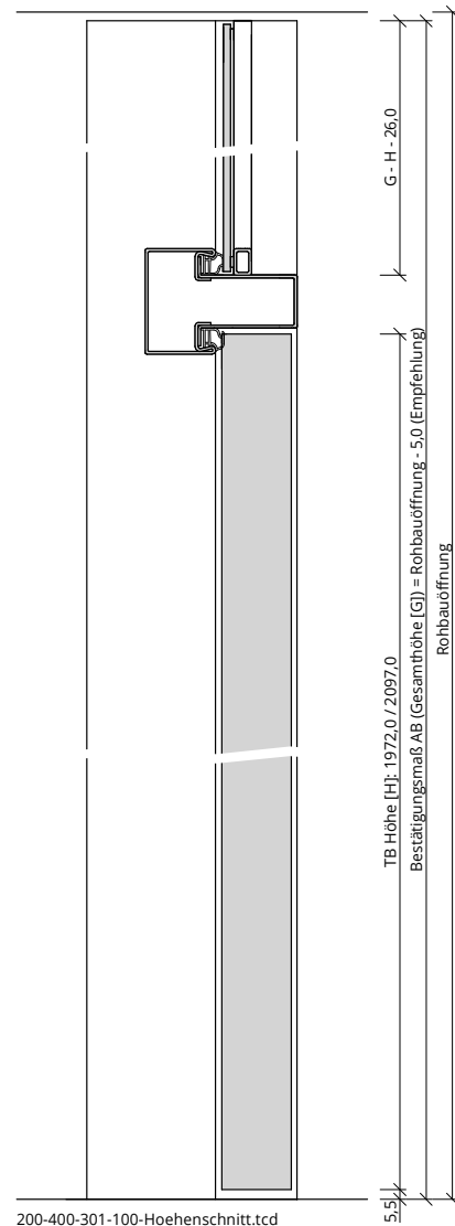
200-400-301-100-Hoehenschnitt.tcd
