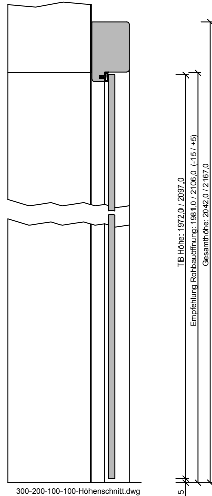
300-200-100-100-Höhenschnitt.dwg
