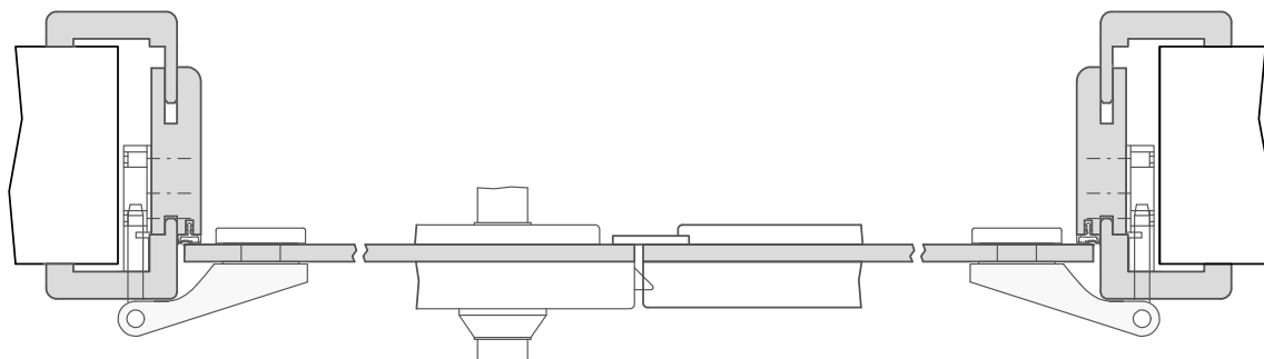
300-100-100-100-Höhenschnitt.dwg
