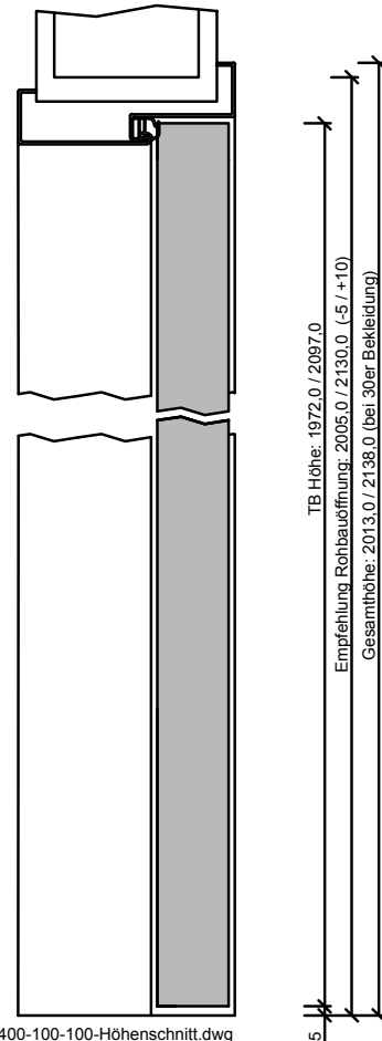
200-400-100-100-Höhenschnitt.dwg
