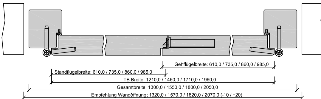
301-108-305-100-Querschnitt.dwg
