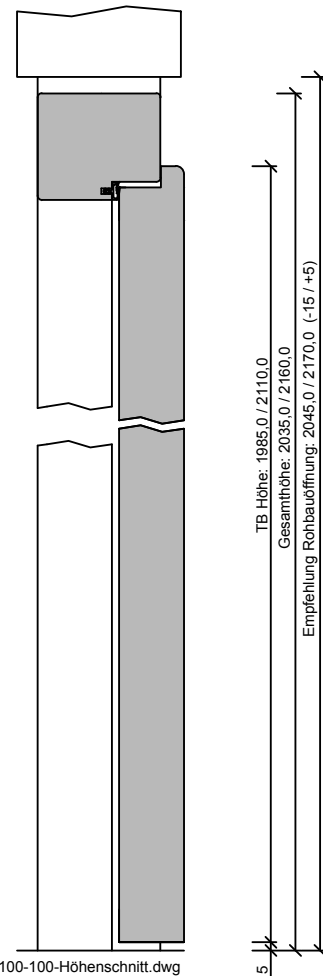
100-300-100-100-Höhenschnitt.dwg
