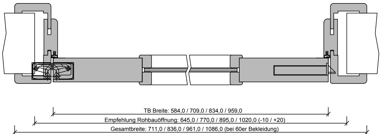
Q-FR-TB-HZ-1FLG-STU-FR-LA.dwg
