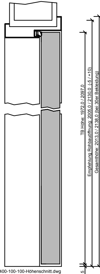
200-400-100-100-Höhenschnitt.dwg
