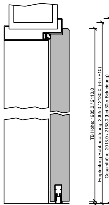
100-400-100-304-Höhenschnitt.dwg
