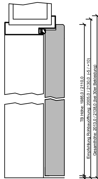
150-440-100-100-Höhenschnitt.dwg
