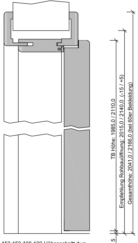
150-150-100-100-Höhenchnitt.dwg
