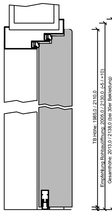
115-411-100-304-Höhenschnitt.dwg
